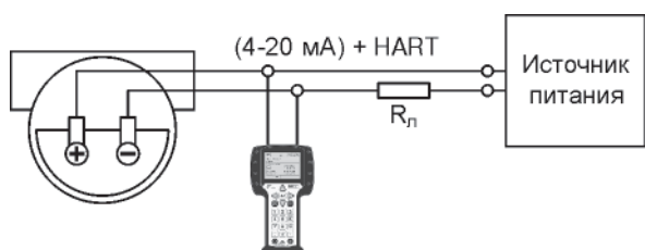
Рис.4. Подключение коммуникатора при R_l > 250 \text{ Ом} .
