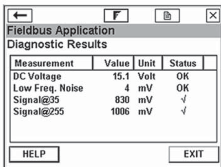
Рис. 2. Диагностика линий Foundation Fieldbus.
