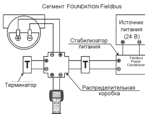
Рис.7. Подключение коммуникатора к сегменту FOUNDATION Fieldbus.
