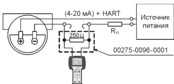
Рис.5. Подключение коммуникатора при R_l < 250 \text{ Ом} .
