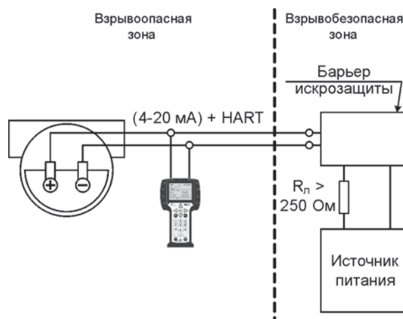
Рис.6. Подключение коммуникатора во взрывоопасной зоне.
